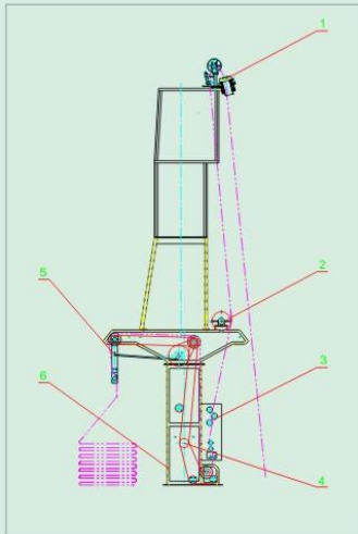
1.退捻装置 2.拍打装置 3.开幅对中装置 4.电气传动部件 5.落布装置 6.机体机架部件 1.untwisting device 2.beating device 3.Open width centering device 4.Electrical transmission parts 5.plaiting apparatus 6.frame parts
